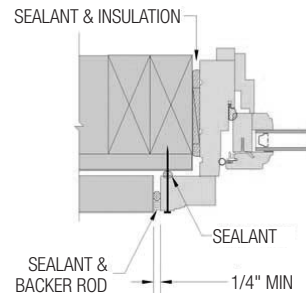
FIG. 18: SIDE JAMB
