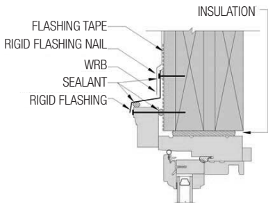
FIG. 14: HEAD JAMB
